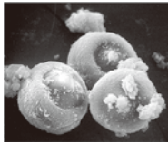
都市部のスギ花粉(直径約30μm)に付着する大小の微粒子
